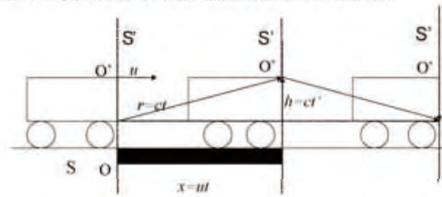
用光子由車廂地板射向天花板，略加修改愛因斯坦的思想實驗。
